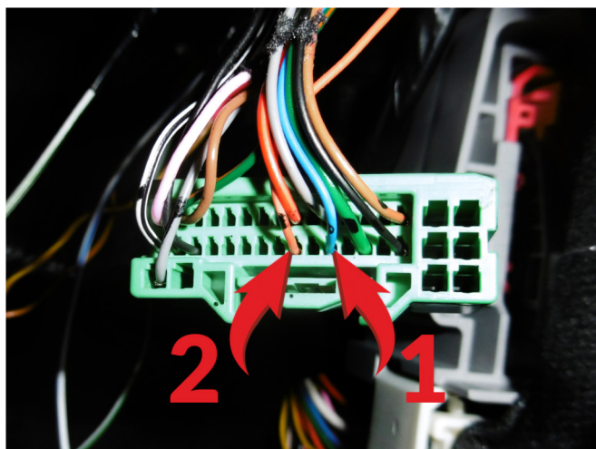
1 - Зажигание 1 (синий провод); 2 - Зажигание 2 (оранжевый провод)
