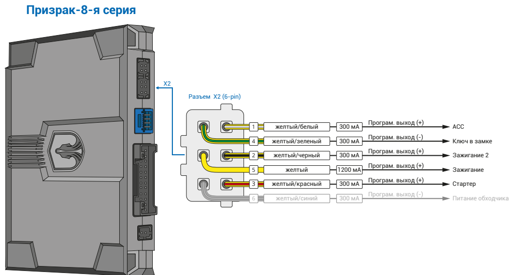
Рис.3 Подключение выходов автозапуска
