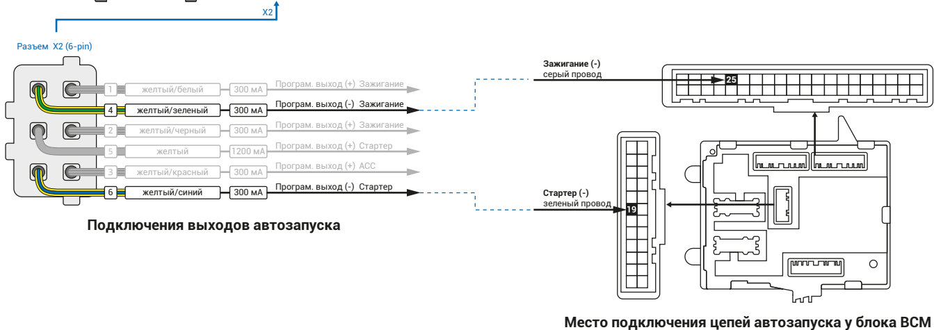
Рис.4 Схема подключения автозапуска
