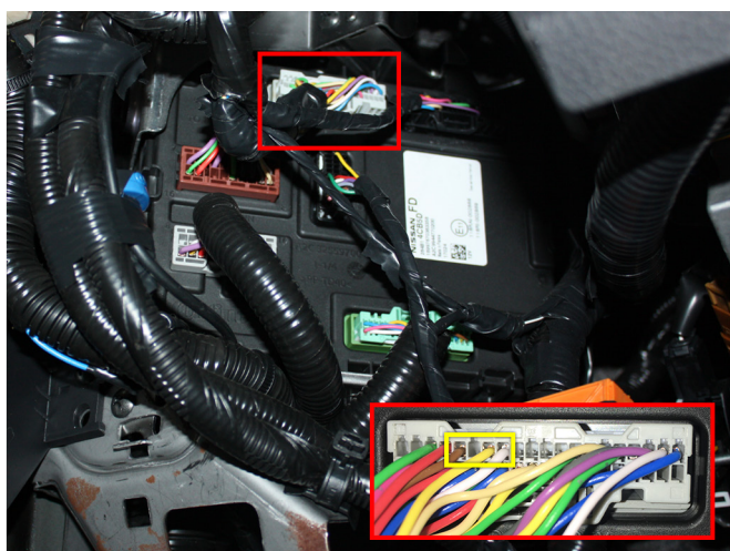
Подключение к цепи: Зажигание - (контакты №25, 27, 28)
