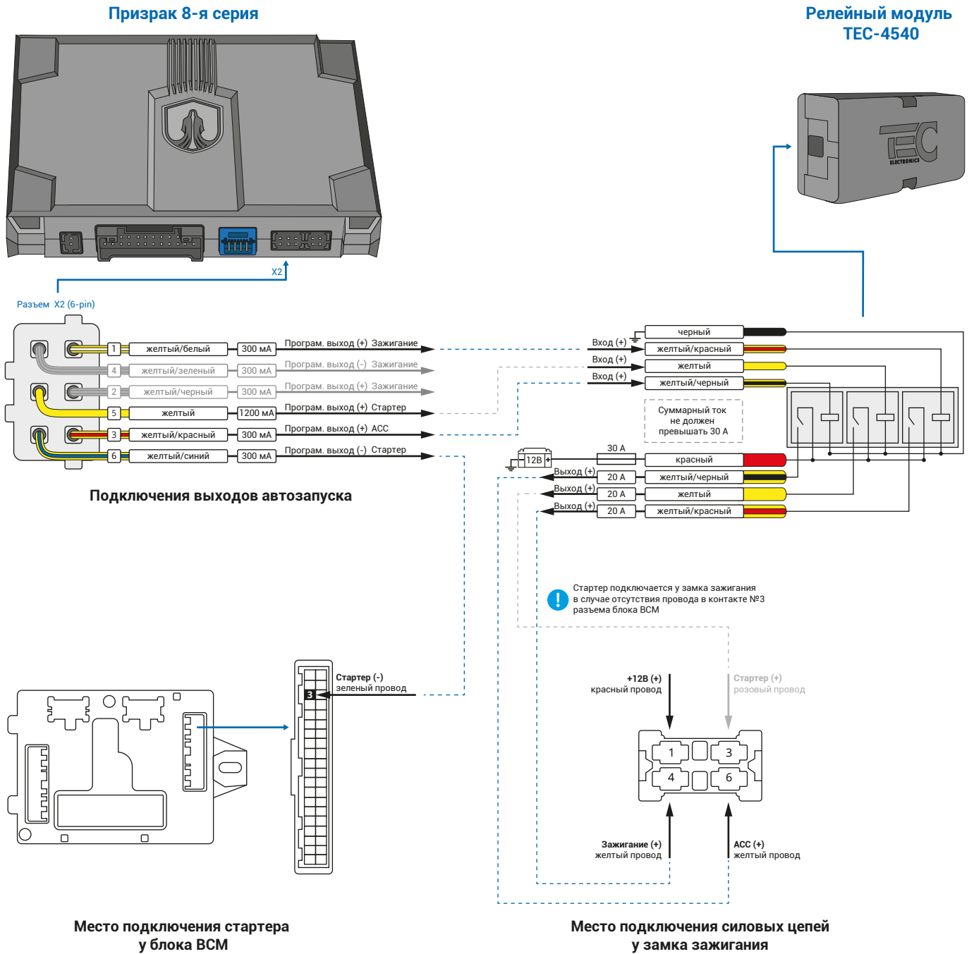
Рис.2 Схема подключения автозапуска
