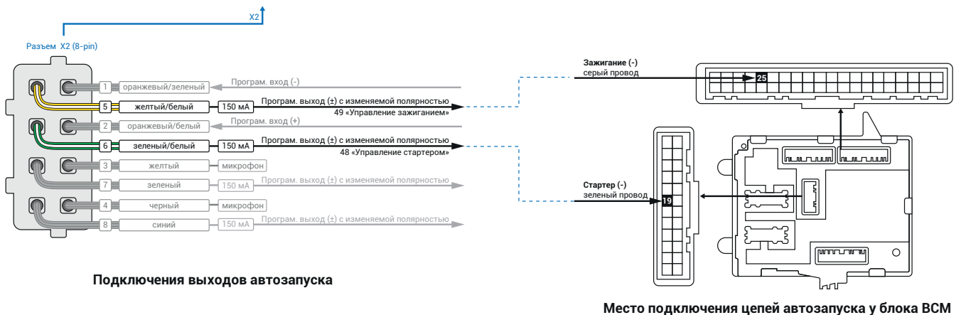
Рис.4 Схема подключения автозапуска
