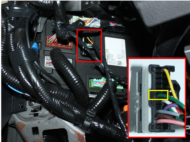
Рис.2 Подключение стартера
