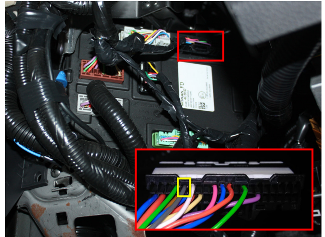
Рис.3 Подключение цепей автозапуска
