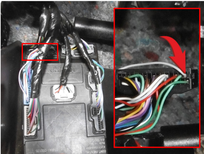
Подключение Зажигание 2 (серый провод, контакт №32)
