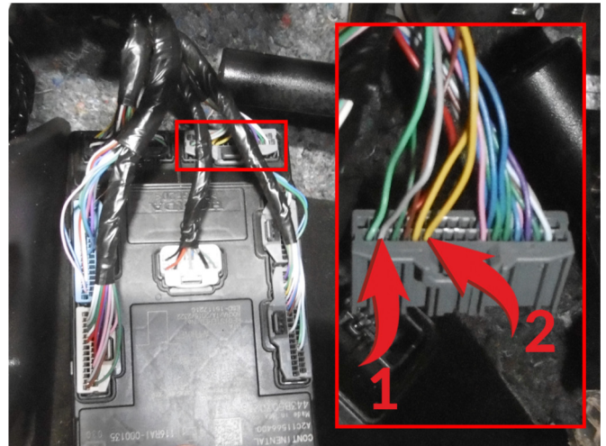
Подключение к цепям запуска двигателя: 1 – Зажигание 1 (серый провод, контакт №2); 2 – Стартер (желтый провод, контакт №6)
