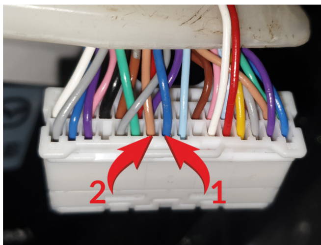
Подключение к цепям запуска: 1 – Зажигание + (синий провод); 2 – Стартер + (коричневый провод).
