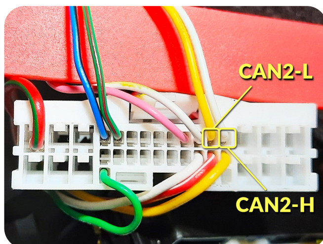
CAN2-H – белый провод, контакт № 13; CAN2-L – желтый провод, контакт № 12.
