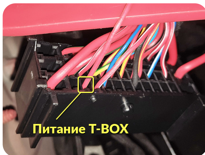
Питание T-BOX – красно-желтый провод, контакт № 29
