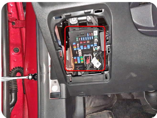
Подключение в черном 39-контактном разъеме монтажного блока слева от рулевой колонки
