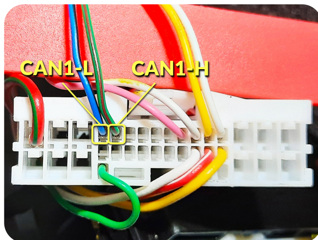
CAN1-H – зелено-красный провод, контакт № 5; CAN1-L – сине-черный провод, контакт № 4.
