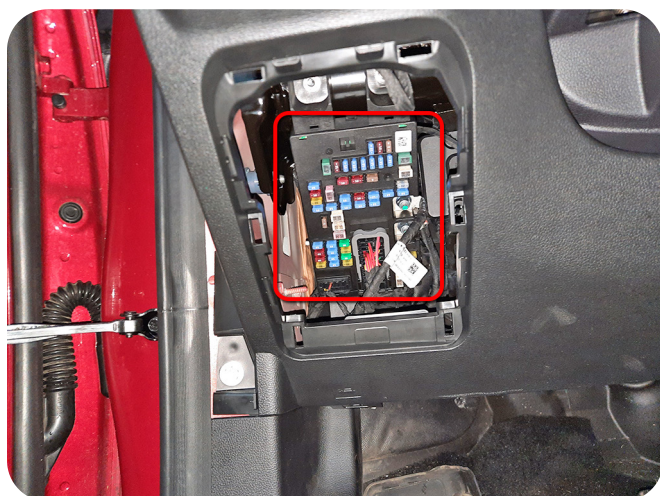
Подключение в черном 39-контактном разьеме монтажного блока слева от рулевой колонки
